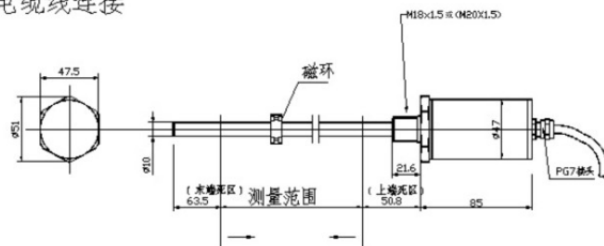
电缆线连接
